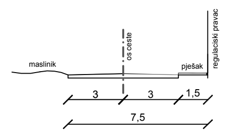
KARAKTERISTIČAN POPREČNI PRESJEK JAVNE PROMETNICE B - B M 1:200
