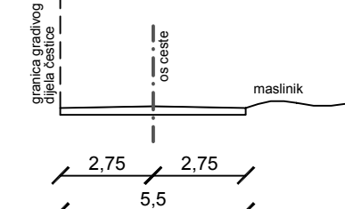
KARAKTERISTIČAN POPREČNI PRESJEK JAVNE PROMETNICE B - B M 1:200
